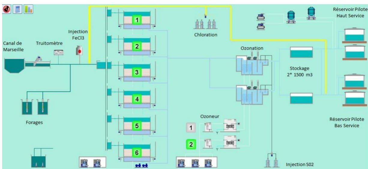
Figure 6: Les étapes de la production d'eau potable -Synoptique de l'usine de potabilisation.
